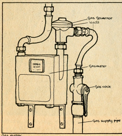
Gas meter
